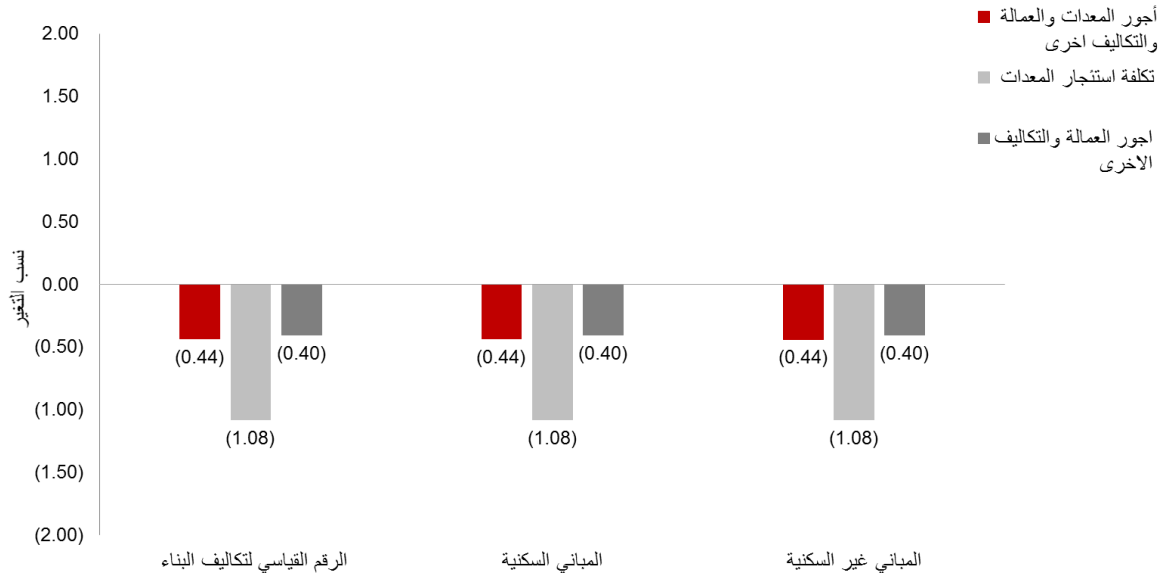
شكل (3) | نسب التغيير في الأرقام القياسية لأجور المعدات والعمالة والتكاليف الأخرى - النصف الأول 2016
