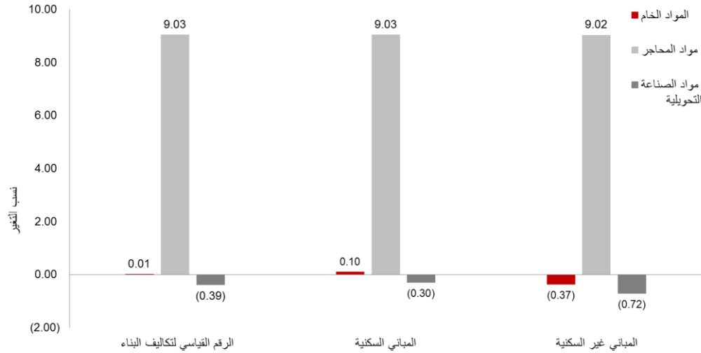
شكل (2) | نسب التغير في الأرقام القياسية للمواد الخام حسب نوع المبنى - النصف الأول 2016
