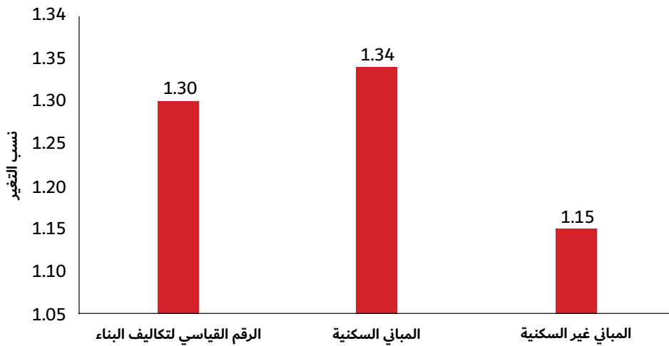
شكل (1) | نسب التغير في الأرقام القياسية لتكاليف البناء لعام 2017
